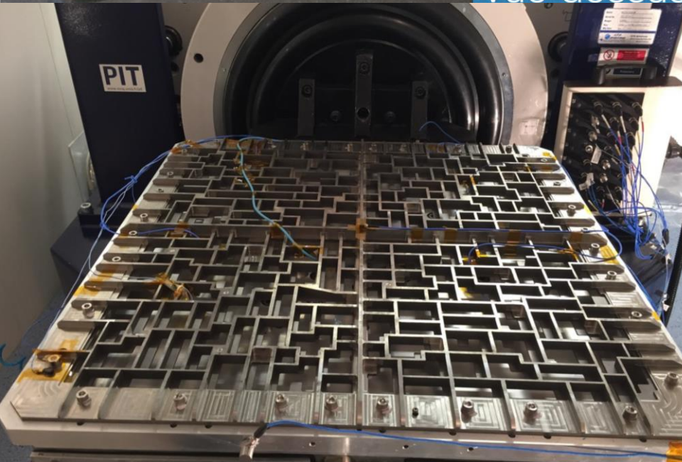
Le masque sur le pot vibrant (sollicitations horizontales et verticales)
